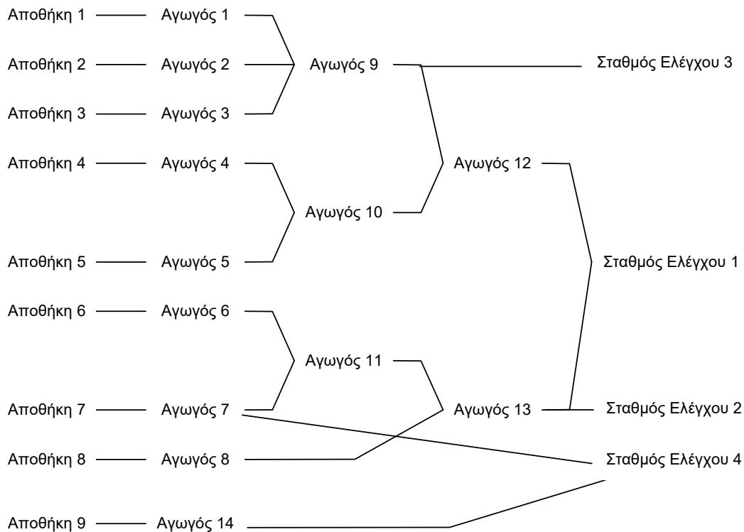
Σχήμα 11.1: Διάγραμμα συστήματος αποχέτευσης εργοστασίου.
